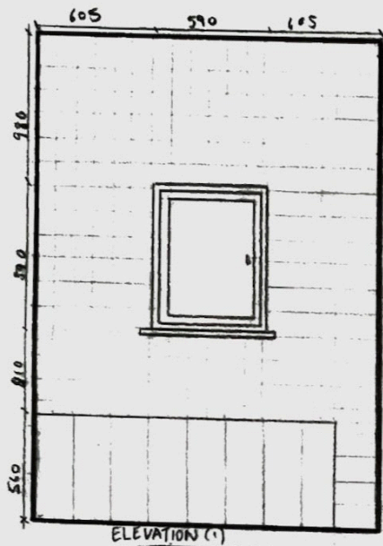
ELEVATION (1)
