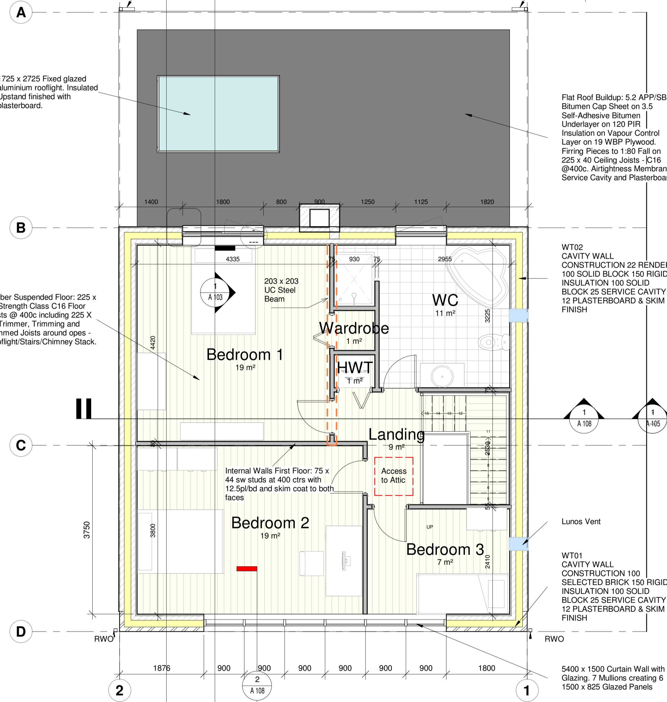
2 2 First FFL 1 : 50
